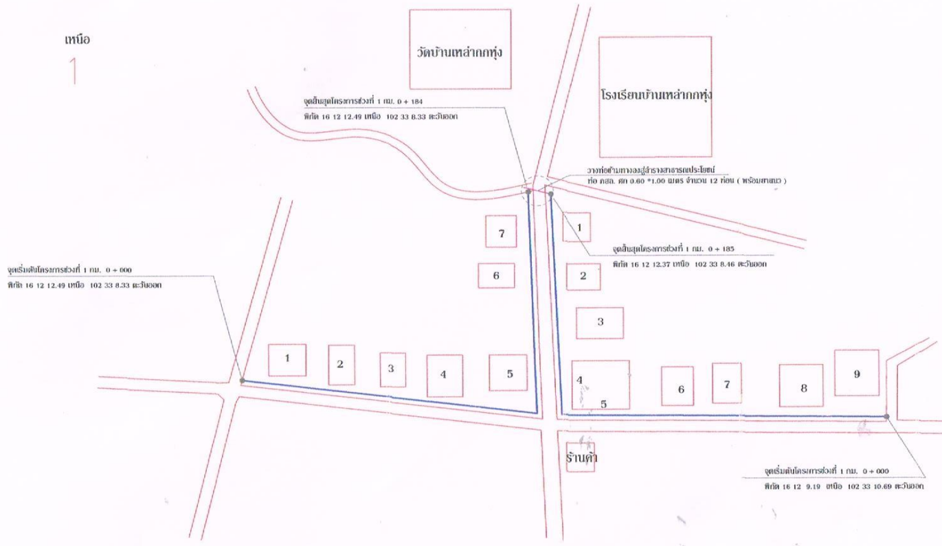
จุดวางท่อคอนกรีตเสริมเหล็ก คก.0.40*1.00 เมตร ช่วงที่ 1 จำนวน 35 ท่อน
